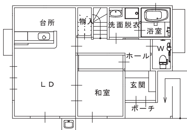
1 階平面図
