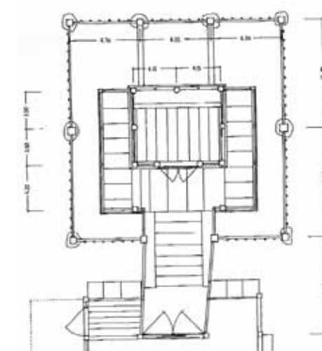
（本殿平面図）
