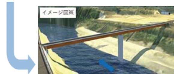
橋梁形式：鋼2径間連続鋼床版桁橋
