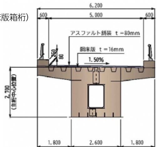
桁横断図
