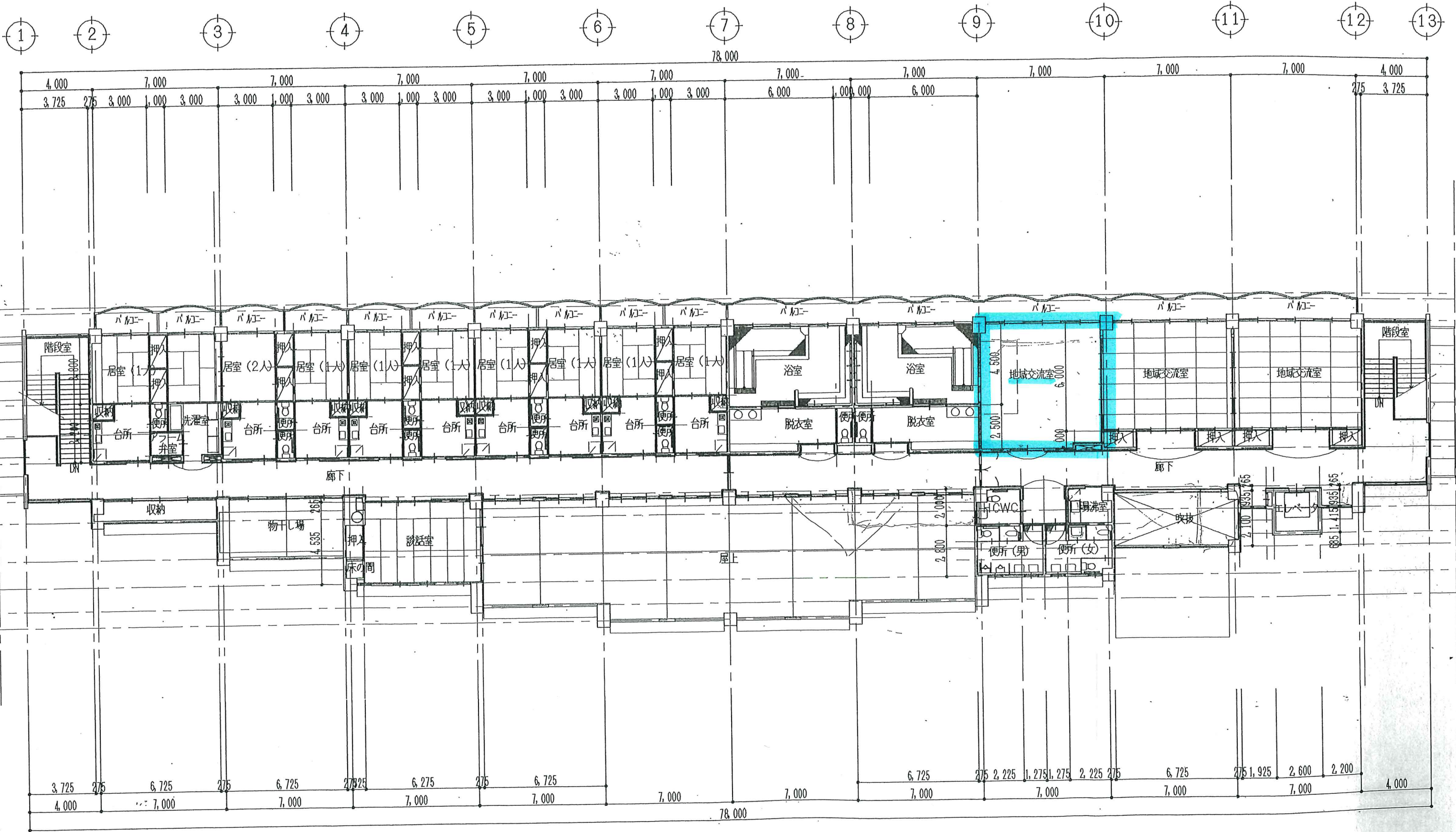
2階平面図 1:200
