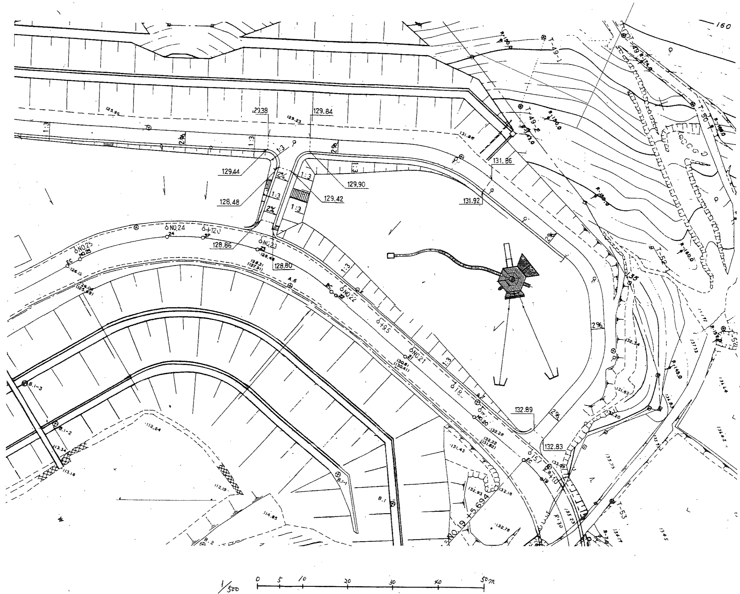
球磨村総合運動公園（遊具広場敷地）平面図
