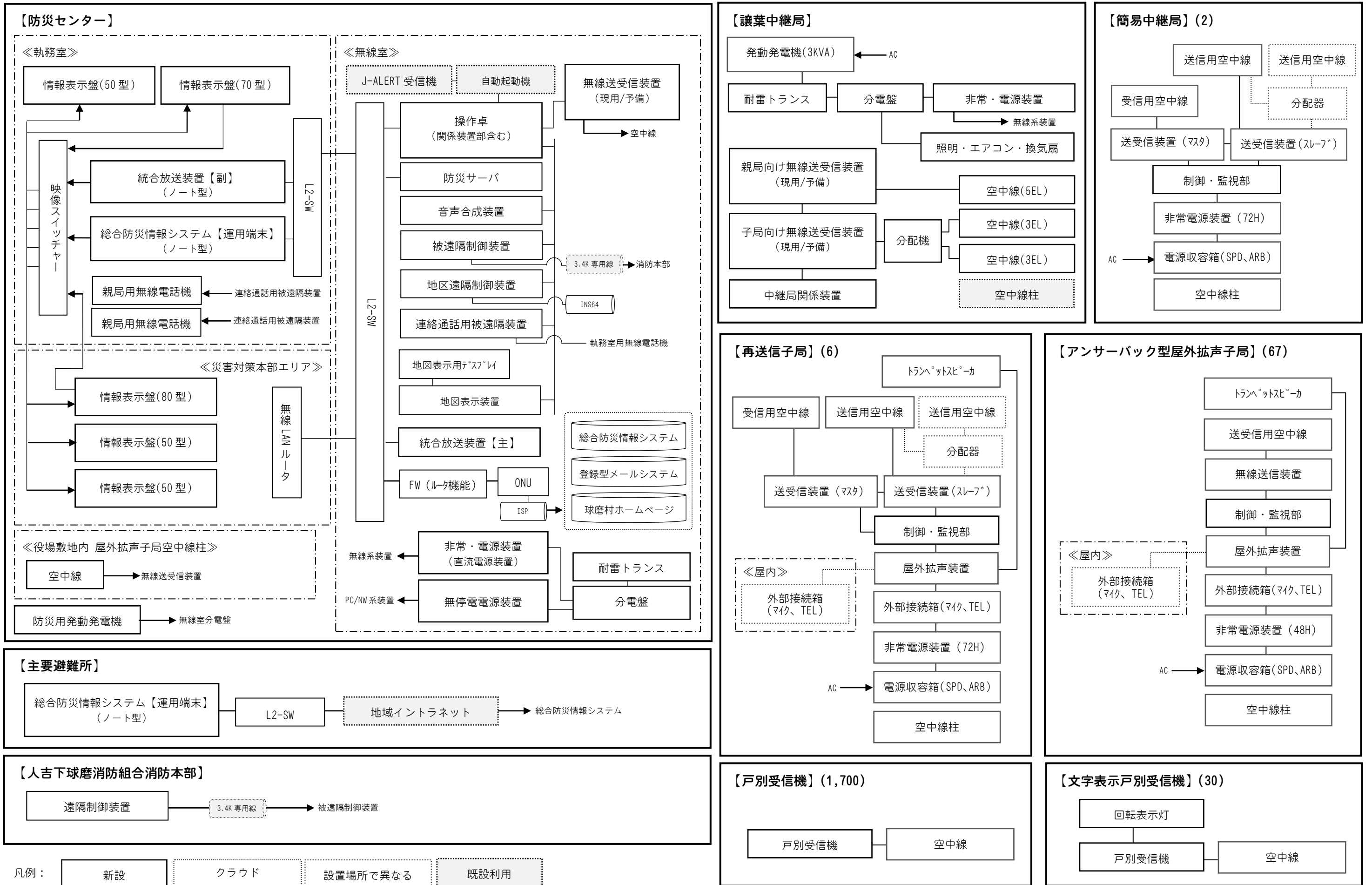
◆球磨村デジタル防災行政無線（同報系）施設整備工事 システム構成図
